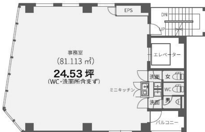
2-11 階平面図
