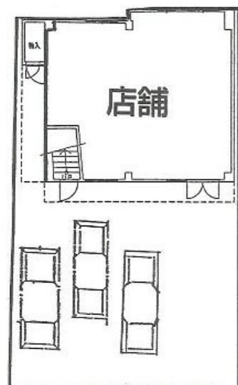
1階平面図
